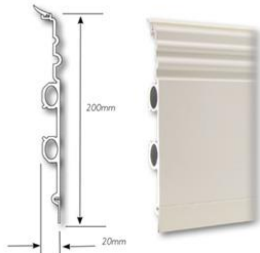
Szuper vékony 20mm-es profilok akár 6m hosszúk
